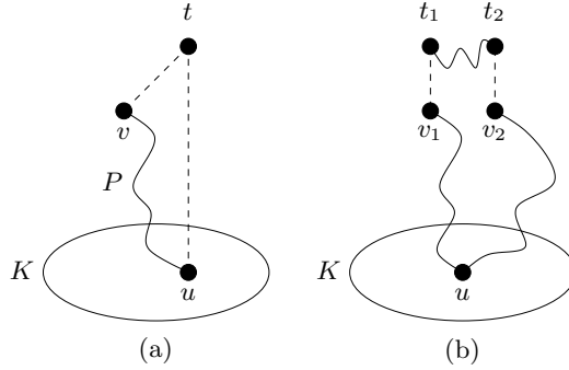
Fig. 4. (a) A t^* -dangerous vertex v . (b) A t_1 -dangerous vertex v_1 and a t_2 -dangerous vertex v_2 .
