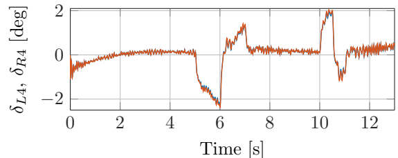
Fig. 12. Control signals: \delta_{L4} (—), \delta_{R4} (—);
